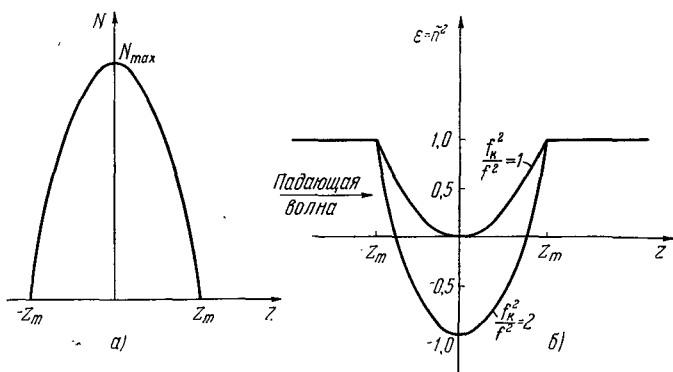
Рис. 17,2. Параболический слой: а) N(z) ; б) \epsilon(z) при \frac{f_K}{f^2} = 1 и \frac{f_K}{f^2} = 2 .
