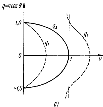
Рис. 29,4. Функции q_{1,2}(v) при распространении в плоскости магнитного меридиана для случая, когда вектор \mathbf{H}^{(0)} направлен под углом \chi = 45^\circ к вертикали (оси z ): а) \theta_0 = 10^\circ , u = \frac{1}{4} ; б) \theta_0 = 0 , u = \frac{1}{4} .
