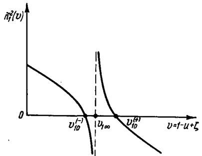
Рис. 27,3. Функция \tilde{n}_1^2(v) при \alpha = \frac{\pi}{2} .
