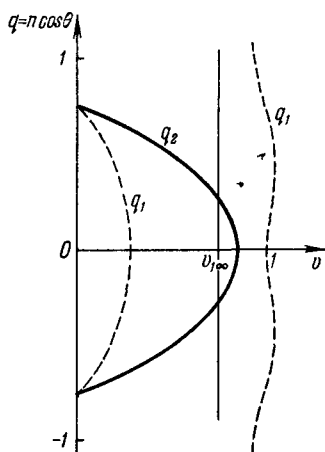
Рис. 29,3. Функции q_{1,2}(v) для распространения на экваторе в плоскости магнитного меридиана
