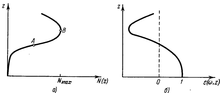
Рис. 30,4. Произвольный плавный слой с одним максимумом.
