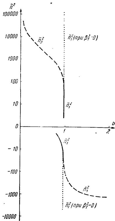
Рис. 12,13. Функции \tilde{n}_1^2 и \tilde{n}_3^2 при u=2 , \alpha=10^\circ и \beta_T^2=10^{-4} .
