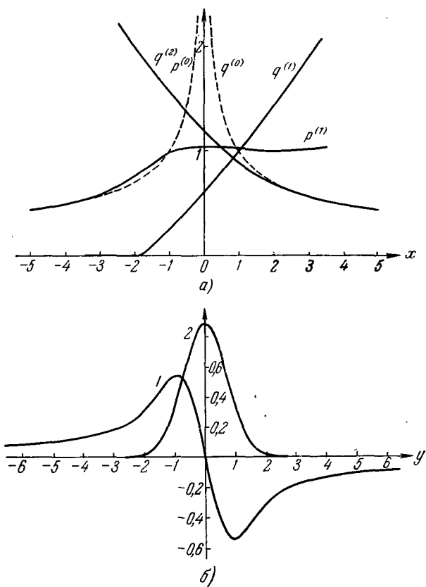
Рис. 12,6. Распространение необыкновенной волны вдоль магнитного поля ( \alpha=0 ) в области резонанса ( u = \frac{\omega H}{\omega^2} \sim 1 ) при отсутствии столкновений ( s = \frac{v_{\text{эф}} \Phi \Phi}{\omega} = 0 ).
