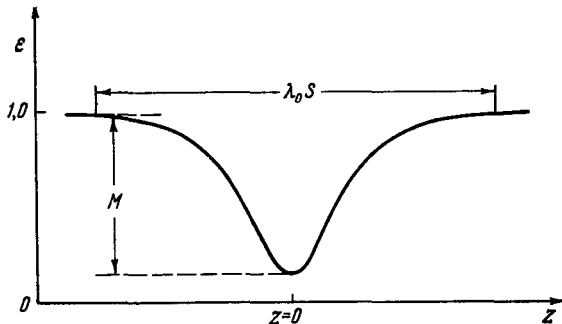
Рис. 18,1. «Симметричный» слой.
