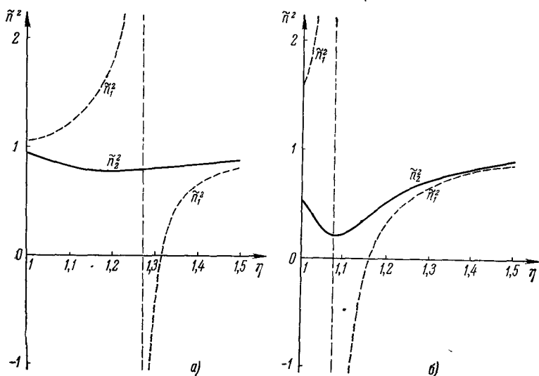
Рис. 36.5. Функции \tilde{n}_{1,2}^2(\eta) в корональной плазме при \alpha=0 (вертикальные пунктирные линии отвечают точке v_{1\infty} ): а) H_b = 2,5 \cdot 10^3 ; б) H_b = 2,5 \cdot 10^2 .
