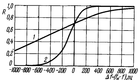
Рис. 33,1. Коэффициент отражения |R| \equiv R для параболических слоев с полутолщиной z_m = 20 км (кривая 1) и 100 км (кривая 2) при отсутствии поглощения.
