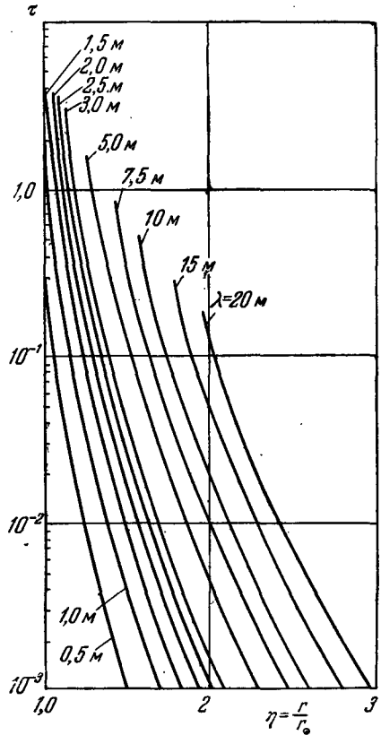
Рис. 36,1. Оптическая толщина короны для радиоволн, распространяющихся по радиусу в направлении к поверхности Солнца. Температура короны T = 10^6 °К. Электронная концентрация распределена согласно формуле (36,1).
