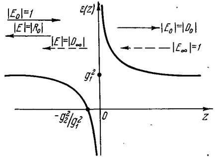
Рис. 27,2. Слой \epsilon(z) = g_1^2 + \frac{g_2^2}{z} .
