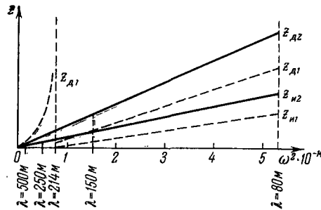
Рис. 35,5. Действующая высота отражения z_{д} и истинная высота отражения z_{и} для линейного ионосферного слоя в зависимости от частоты \omega . Пунктир относится к волне типа 1, а сплошные линии — к волне типа 2.
