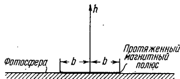
Рис. 36,4. Протяженный магнитный полюс, имеющий форму окружности с радиусом b и находящийся на уровне фотосферы.
