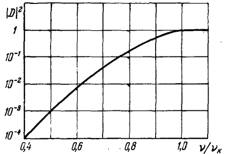
Рис. 28,8. Коэффициент пропускания |D|^2 как функция \frac{v}{v_K} при u = \frac{1}{4} и \omega = 1,76 \cdot 10^7 ( \lambda_0 = 107 м).
