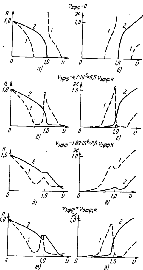
Рис. 11,13. Показатели преломления и поглощения для \lambda_0 = 80 м и различных значений v_{эфф} (значения \alpha и \omega_H указаны в тексте; пунктир относится к волнам типа 1, сплошные линии — к волнам типа 2).
