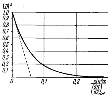
Рис. 28,7. Коэффициент пропускания |D|^2 как функция от \frac{\sin^2 \alpha}{\left(\frac{dN}{dz}\right)_{v=1}} при u = \frac{1}{4} и \omega = 1,76 \cdot 10^7 ( \lambda_0 = 107 м). Сплошная кривая |D|^2 = e^{-2\delta_0} , пунктирная кривая |D|^2 = 1 - 2\delta_0 .
