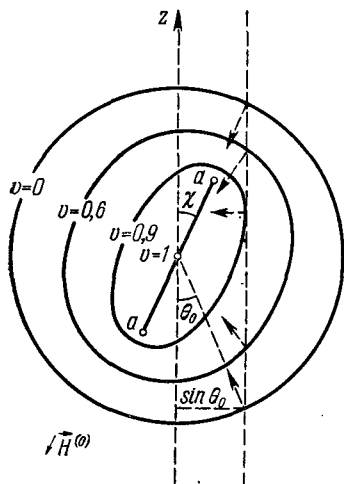
Рис. 29,13. Показатель преломления n_2 для обыкновенной волны в зависимости от угла \theta и параметра v (H^{(0)} = 0,5 \text{ эрст}, \alpha = 25^\circ, \lambda_0 = 80 \text{ м}) .
