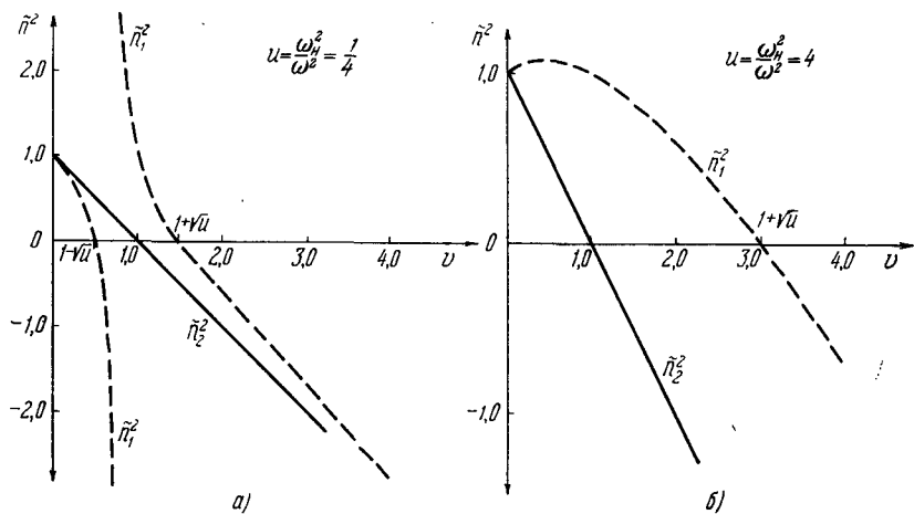
Рис. 11,3. Функции \tilde{n}_{1,2}^2(\nu) при u = \text{const} в случае поперечного распространения (т. е. при \alpha = 90^\circ ): а) u < 1 ; б) u > 1 .
