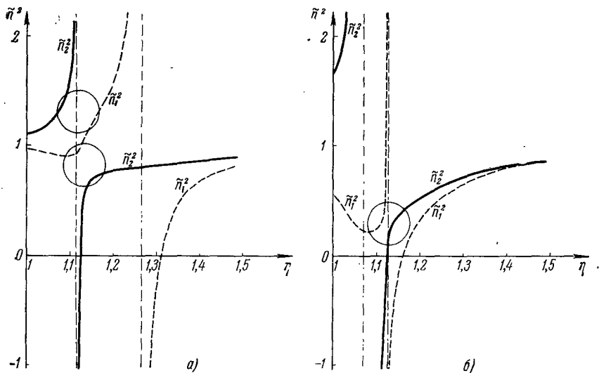
Рис. 36.6. Функции \tilde{n}_{1,2}^2(\eta) в корональной плазме при \alpha=15^\circ (вертикальные пунктирные линии отвечают точкам v_{1\infty} и v_{2\infty} ): а) H_b = 2,5 \cdot 10^3 ; б) H_b = 2,5 \cdot 10^2 .
